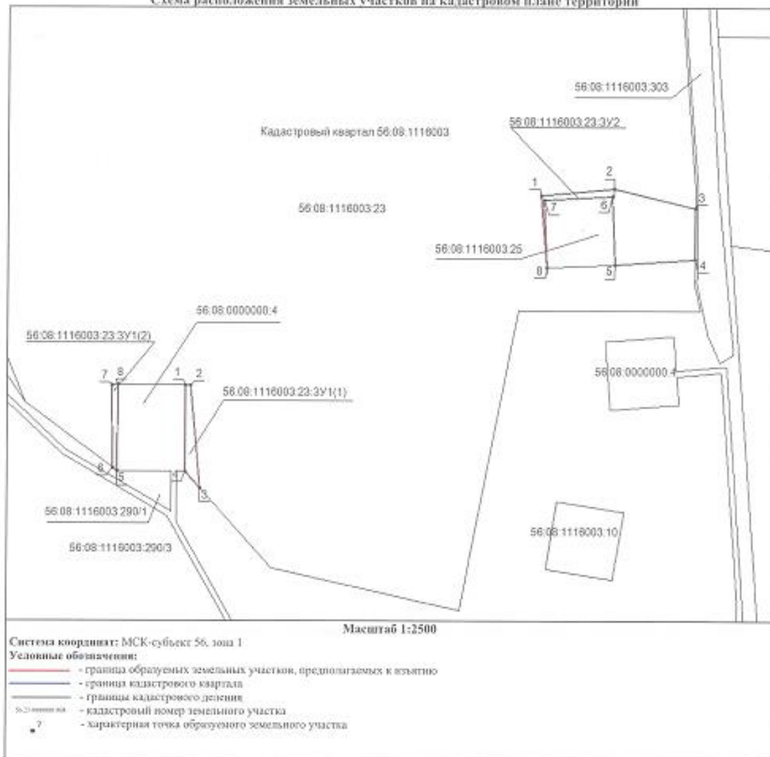
Схема расположения земельных участков на кадастровом плане территории
